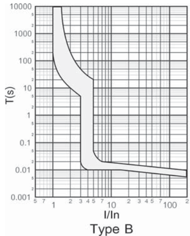
กราฟแสดงคุณลักษณะ เวลา-กระแส ของเซอร์กิตเบรกเกอร์ ชนิด MCB
