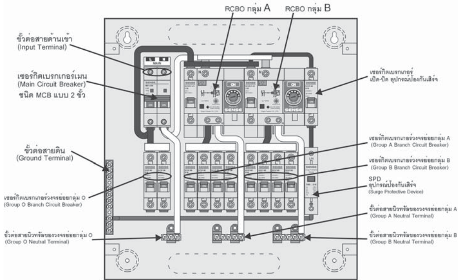
รูปแสดงส่วนประกอบภายในตู้คอนซูมเมอร์ยูนิต รุ่น R2N
