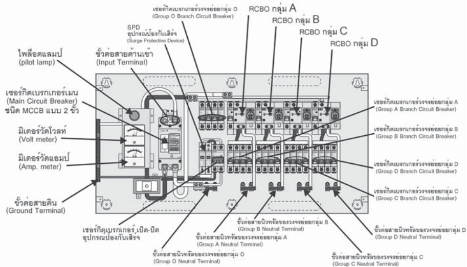
รูปแสดงส่วนประกอบภายในตู้คอนซูเมอร์ยูนิท รุ่น RM4-100
