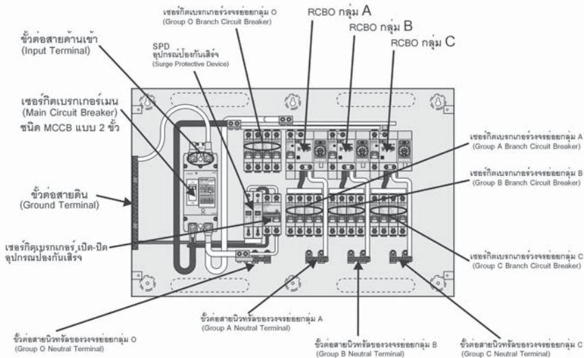
รูปแสดงส่วนประกอบภายในตู้คอนซูเมอร์ยูนิต รุ่น R3-100
